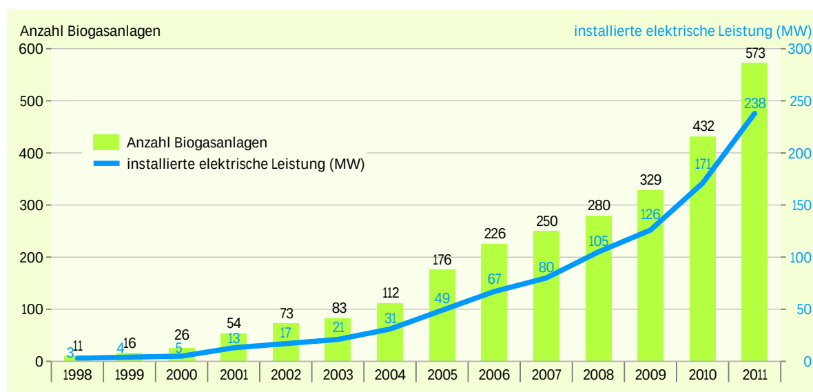
Anzahl und installierte elektrische Leistung der Biogasanlagen in Nordrhein-Westfalen in den Jahren 1998 bis 2011
