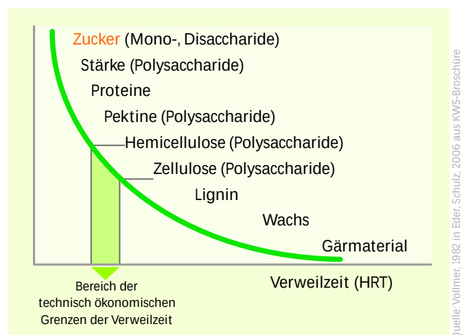
Abbaugeschwindigkeit verschiedener Inhaltsstoffe in Biogasanlagen
